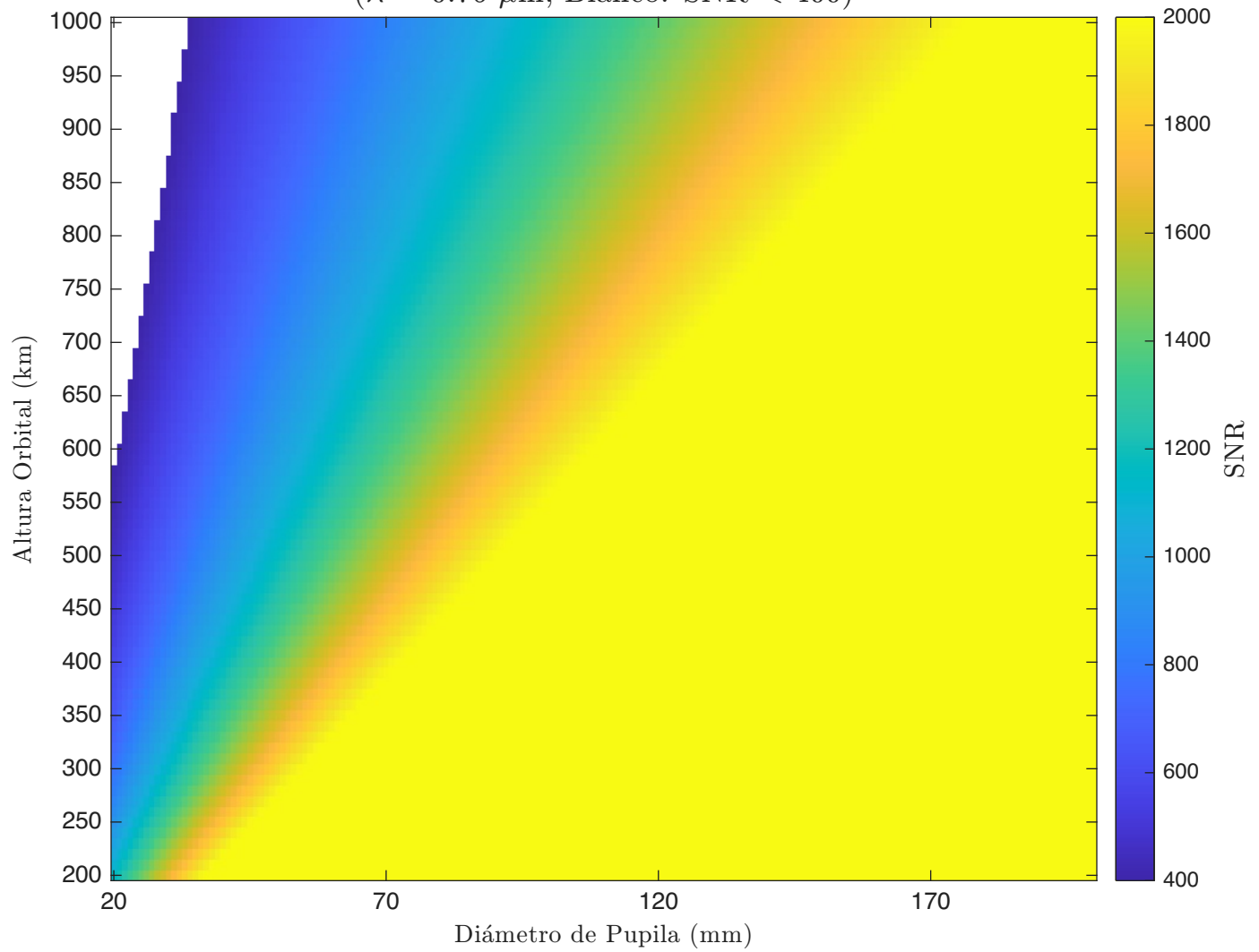
SNR - Korsch - Detector 2 ( \lambda = 0.76 \mu\text{m} , Blanco: SNR < 400)
